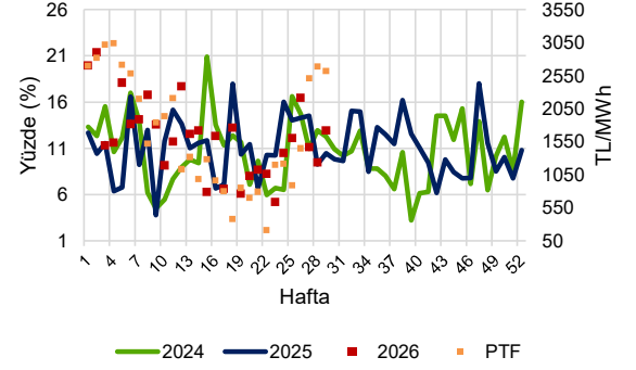
Şekil 11: Doğal Gaz Santralleri Üretiminin Haftalık Bazdaki Payı
