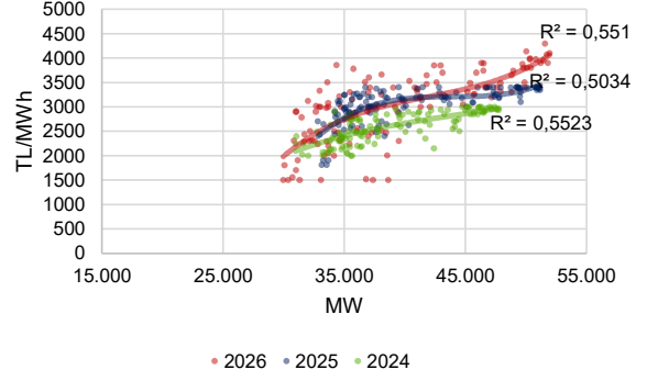
Şekil 15: Hafta İçi Günlere İlişkin PTF-Yük İlişkileri
