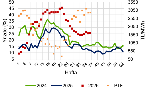
Şekil 10: Kömür Santralleri Üretiminin Haftalık Bazdaki Payı
