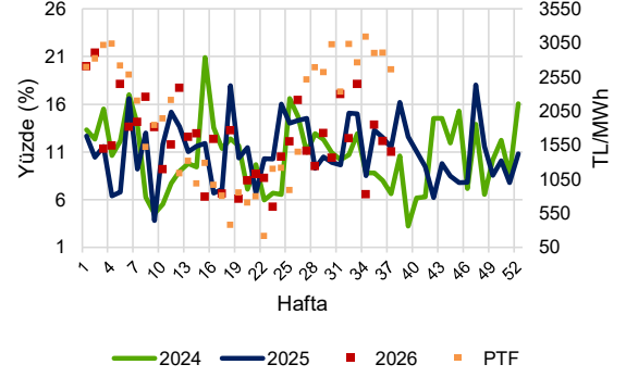
Şekil 11: Doğal Gaz Santralleri Üretiminin Haftalık Bazdaki Payı
