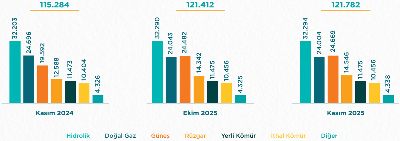
Kaynaklara Göre Kurulu Güç Gelişimi (MWe)
