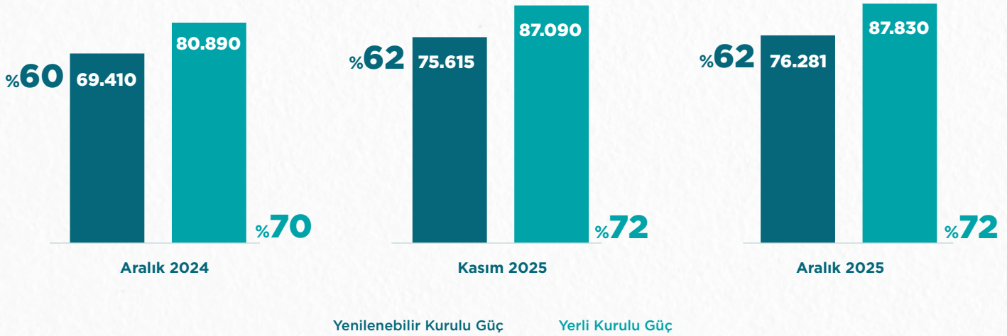
Yerli ve Yenilenebilir Kurulu Güç Gelişimi (MWe)
