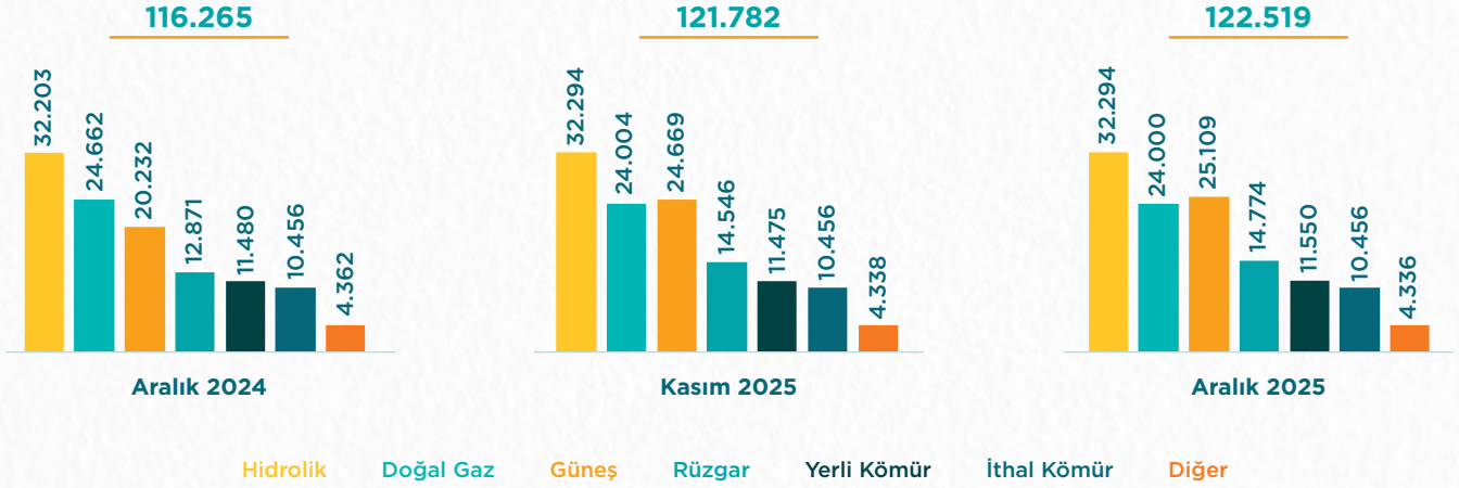
Kaynaklara Göre Kurulu Güç Gelişimi (MWe)
